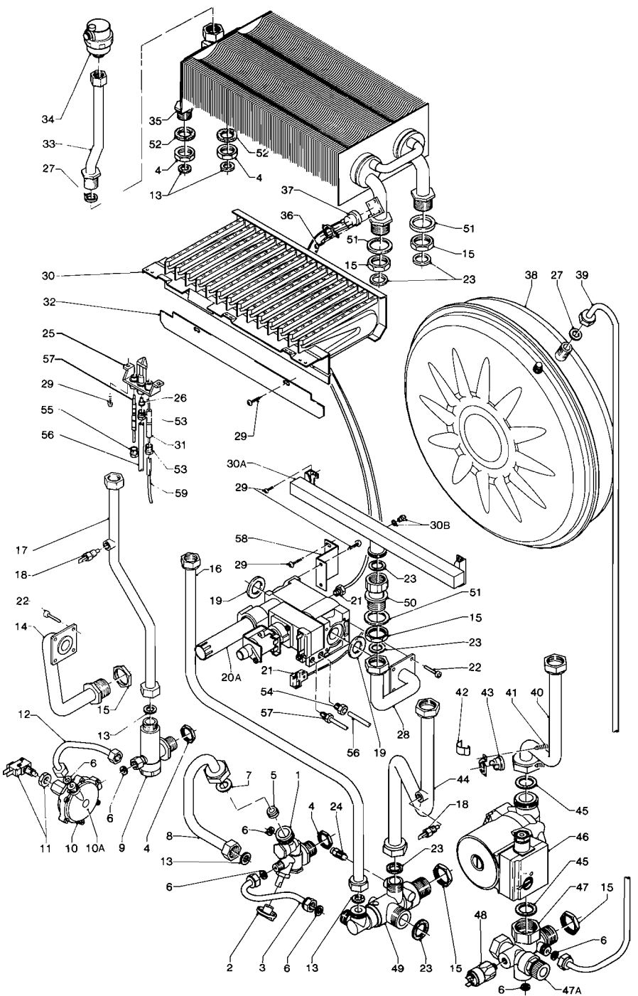
TAV. - DRWG. 2.00 I
