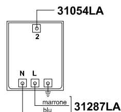
TRASFORMATORE AC1 230VAC 25HZ COD. 88018LA
