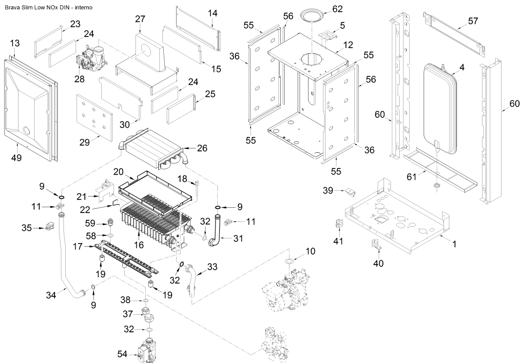
Brava Slim Low NOx DIN - interno
