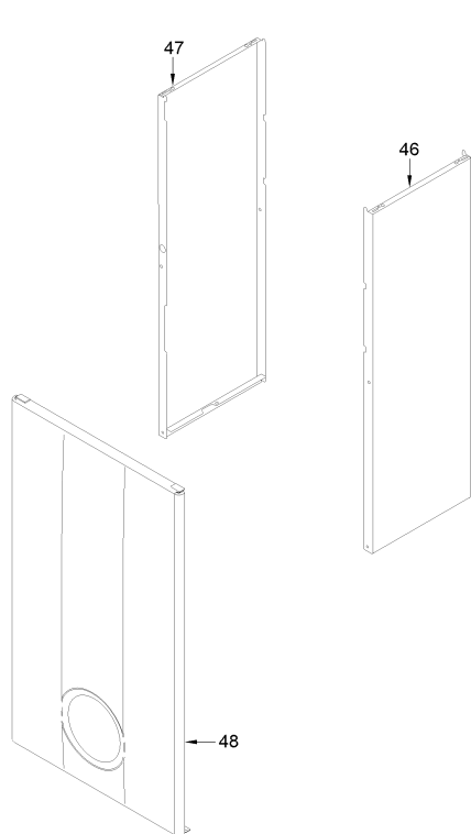
Brava Slim Low NOx DIN - interno
