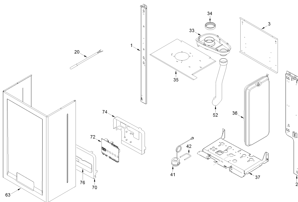
BRAVA DGT HE 12 T - telaio / pannello strumenti
