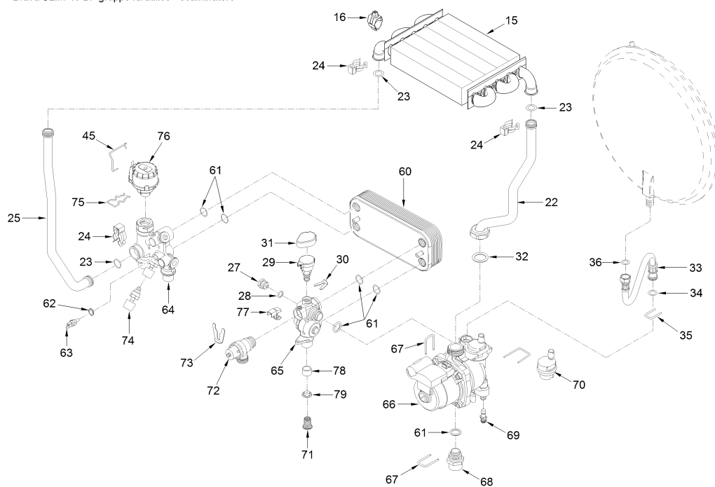
Brava SLIM 40 BF gruppo idraulico - scambiatore
