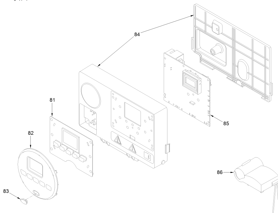
Brava SLIM 40 BF gruppo pannello strumenti
