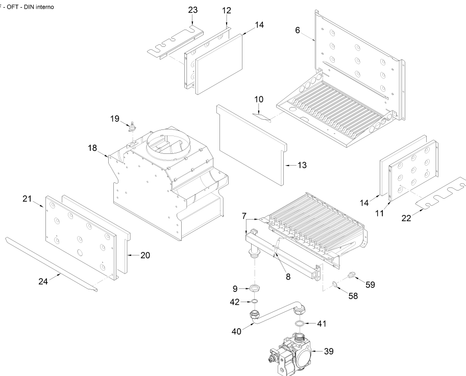
Murelle EV OF - OFT - DIN interno
