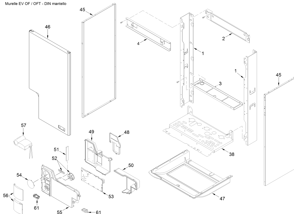
Murelle EV OF / OFT - DIN mantello
