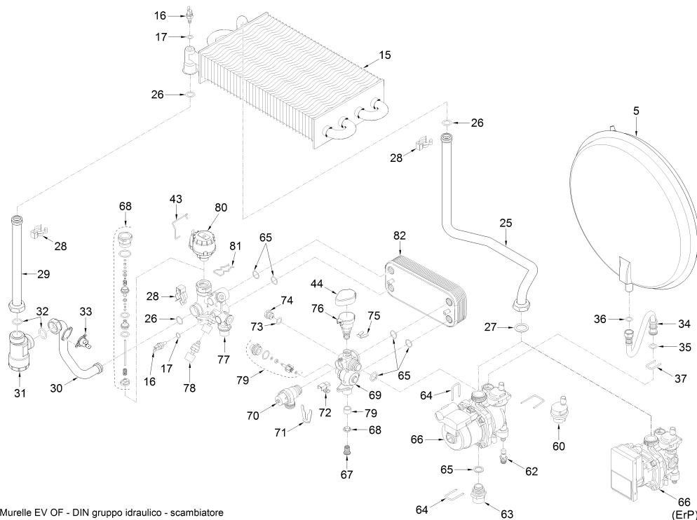
Murelle EV OF - DIN gruppo idraulico - scambiatore
