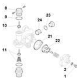
Gruppo distribuzione mandata codice 4364202
